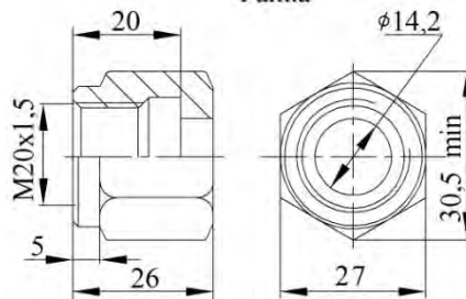
Гайка
