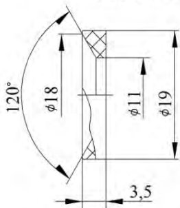
Кольцо ТЖИУ.711171.005
