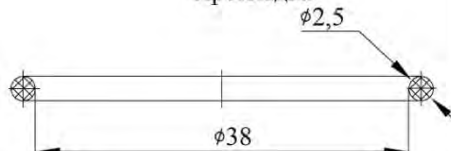
Прокладка
