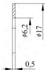
Шайба ТЖИУ.711141.013
